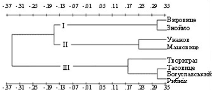
Рис. 2. Дендрограма кореляційних зв'язків провідних петротипів гранітоїдів Дійського масиву за їхнім мікроелементним складом: I – III – породні групи петротипів з додатними значеннями коефіцієнтів кореляції
