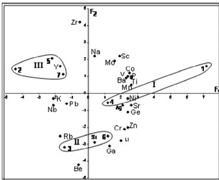
Рис. 3. Факторна діаграма фігуративних точок мікроелементного складу провідних петротипів гранітоїдів Дійського масиву. Назви петротипів гранітоїдних порід за їх номерами див. на рис. 1. Оконтурено породні групи (I – III) петротипів з додатними значеннями коефіцієнтів кореляції, згідно з дендрограмою на рис. 2
