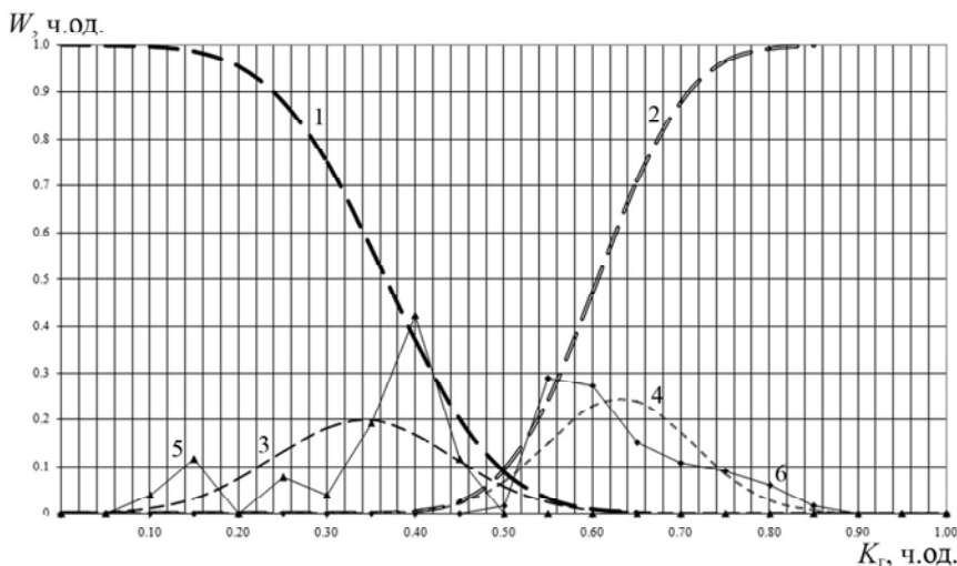
Рис. 5. Криві розподілу для газонасичених і водоносних колекторів: 1 – вода, кумулянта крива; 2 – газ, кумулянта крива; 3 – вода, теоретична крива; 4 – газ, теоретична крива; 5 – вода, фактична крива; 6 – газ, фактична крива.
