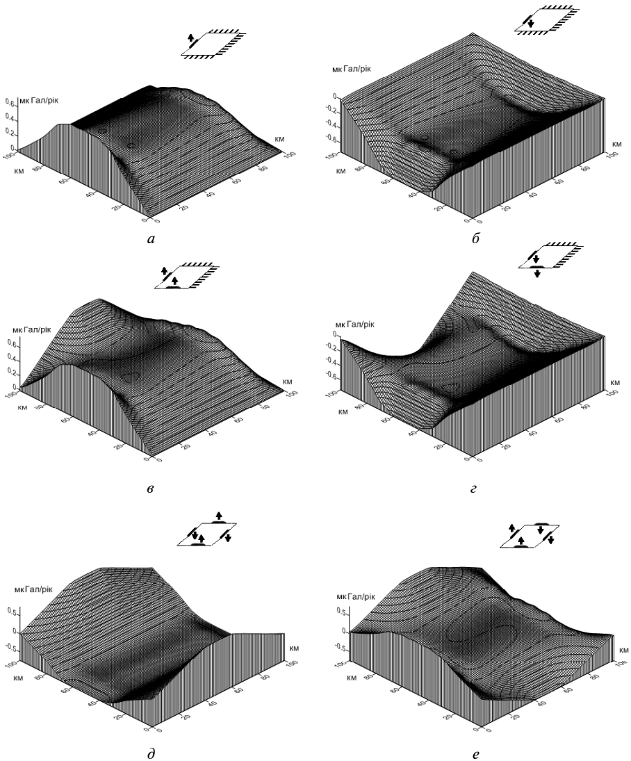
Рис. 2. Розподіли швидкостей змінювання аномального гравітаційного поля в околах сучасних вертикальних рухів мікроблоків кристалічного фундаменту ДДЗ, які розташовані на середині сторін нерухомих блоків: a – мікроблок рухається вгору; б – мікроблок рухається вниз; в – мікроблоки, розташовані на суміжних сторонах блока, рухаються вгору; г – мікроблоки, розташовані на суміжних сторонах блока, рухаються вниз; д – пара мікроблоків, розташована на протилежних сторонах блока, рухається вгору, інша пара – вниз; е – пара мікроблоків, розташована на суміжних сторонах блока, рухається вгору, інша пара – вниз
