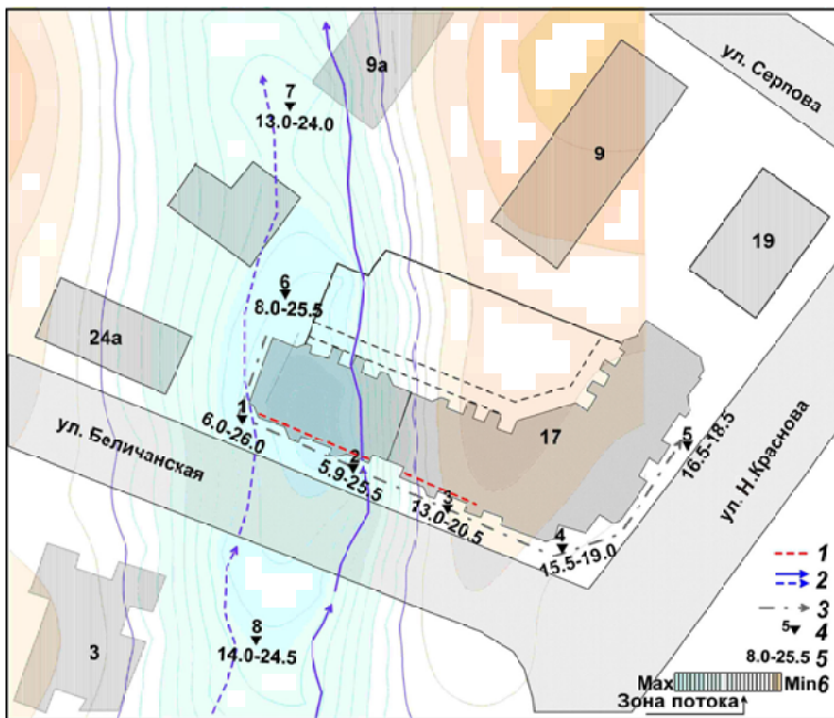
Рис. 4. Карта зон увлажнения грунтов в районе дома № 17 по ул. Н. Краснова (г. Киев): 1 – контур участка образования трещин в стенах дома; 2 – направления миграции грунтовой воды в пределах фильтрационного потока; 3 – профиль георадарного зондирования; 4 – пункт ВЭРЗ; 5 – интервал зоны увлажнения грунтов, м; 6 – шкала относительного увлажнения грунтов
