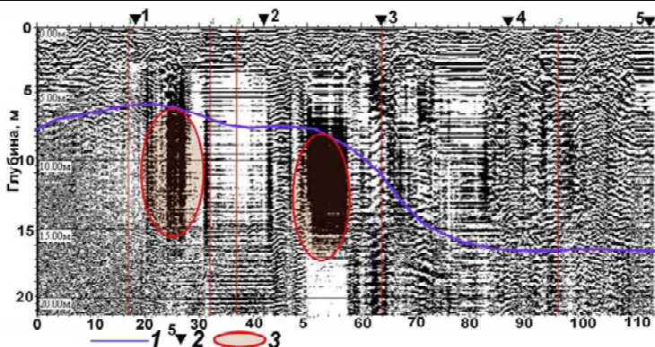
Рис. 5. Вертикальний георадарний розріз вдоволь фасадної частини дому № 17 по ул. Н. Краснова (г. Київ): 1 – рівень ґрунтових вод; 2 – пункт ВЕРЗ; 3 – суффузійно-ослаблена зона
