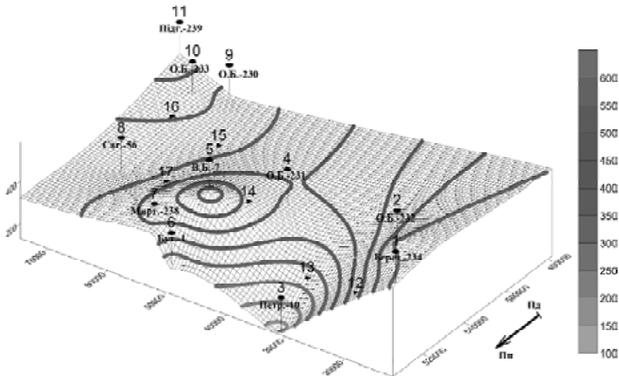
Рис. 4. Район Білоцерківсько-Остап'ївського виступу південного борту і прилеглої частини південної прибортової зони центрального грабену ДДЗ. Тривимірне зображення розподілу поля товщини підсольового СФК девону ( D_{2-3} , м) за даними буріння глибоких свердловин і просторових інтерполяцій за методами Колмогорова та звичайного кригінгу (координати умовні, м). Кругами позначено еталонні точки (свердловини, див. табл. 1), трикутниками – досліджені площі (точки прогнозу, див. табл. 2)
