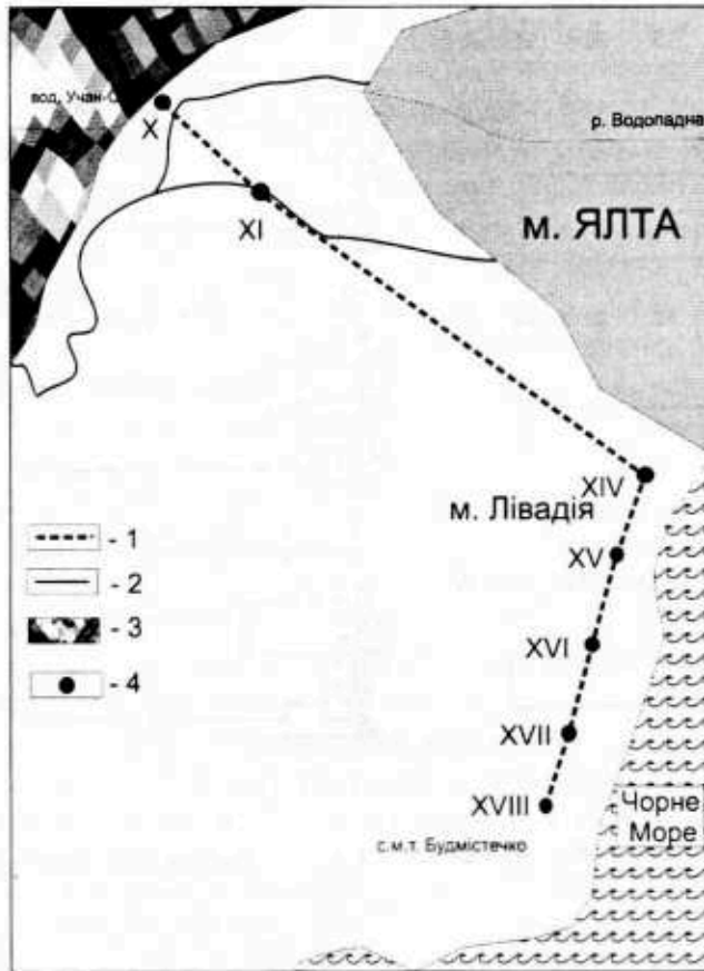
Рис. 1. Картохема висотного профілю (X, XI, XIV) та профілю «Казкова стежка» (XIV–XVIII): 1 – лінії профілю; 2 – дороги на гору Ай-Петрі; 3 – скеляста місцевість; 4 – локалізація ценопопуляцій
