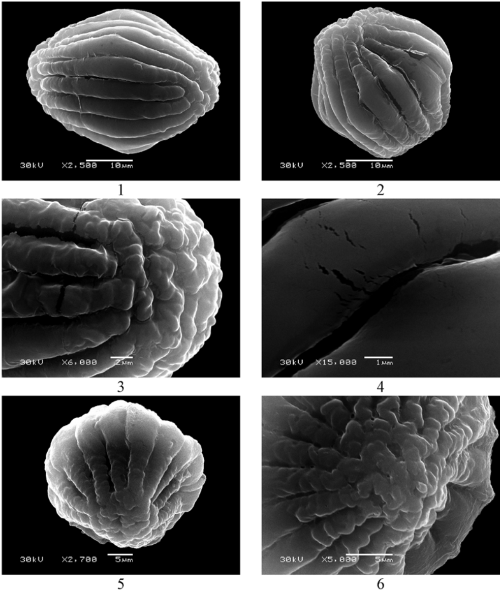
Рис. 2. Пилкові зерна Utricularia (СЕМ): 1–4– U. vulgaris (1, 2 – вигляд з екватора; 3 – скульптура поверхні апокольпумів; 4 – скульптура поверхні мезокольпумів); 5, 6– U. intermedia (5 – вигляд з полюса, 6 – скульптура поверхні апокольпумів)
