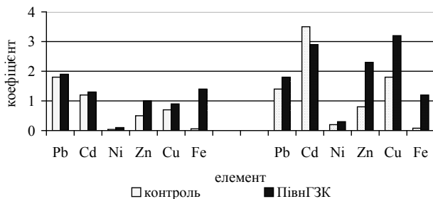
Рис. 2. Транслокаційні коефіцієнти деяких елементів у H. lilioasphodelus і H. middendorffii в контролі і за умов забруднення Fig. 2. Translocation coefficients of some elements in H. lilioasphodelus and H. middendorffii in control and under conditions of contamination
