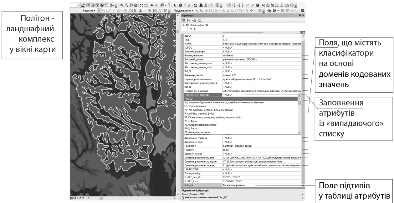
Рис. 2. Використання доменів для заповнення таблиці атрибутів ландшафтної карти України: вибір значення із «випадаючого» списку (ПЗ ArcGISforDesktop)
