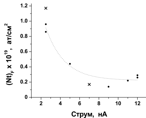
Рис. 4. Залежність кількості атомів фтору в поверхневому шарі кремнію від величини струму альфа-частинок: ● – зразок № 1; × – зразок № 2
