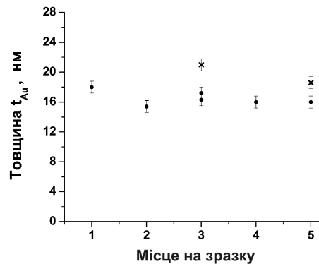
Рис. 3. Залежність товщини поверхневого шару золота від місця на робочій поверхні зразка: ● – зразок № 1; × – зразок № 2. Місця для вимірів розташовувалися вздовж лінії, яка проходила через центр зразка (місце 3). Місця 1 і 5 вибиралися на краях зразка
