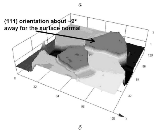
Рис. 3. Сукупні дані методу EBSD і лазерної профілометрії. Двовимірні ( a ) та тривимірні ( б ) зображення поверхні полікристалічного вольфрамового дзеркала після розпилення 4 мкм (у середньому, як знайдено за втратою маси) іонами аргону з енергією 600 еВ [5]. Найвищі зерна мають відхилення \approx 9^\circ від нормального положення грані (111)
