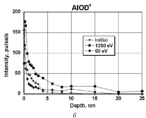
Рис. 11. Дані ВІМС аналізу щодо складу приповерхневого шару Al дзеркал. Показані дані виходу іонів AlO^- та AlOD^+ залежно від глибини їх знаходження [20]
