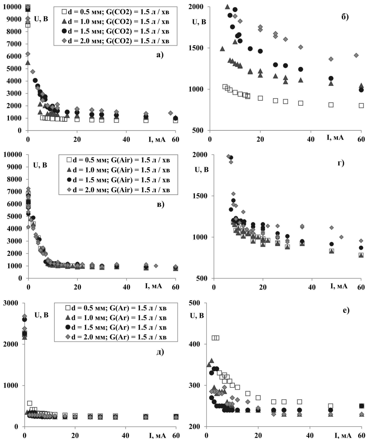
Рис. 5. Виміряні вольт-амперні характеристики в потоках G = 1,5 л/хв: \text{CO}_2 (а, б), повітря (в, г) та \text{Ar} (д, е) за використання різних d та позитивній полярності високовольного електрода
