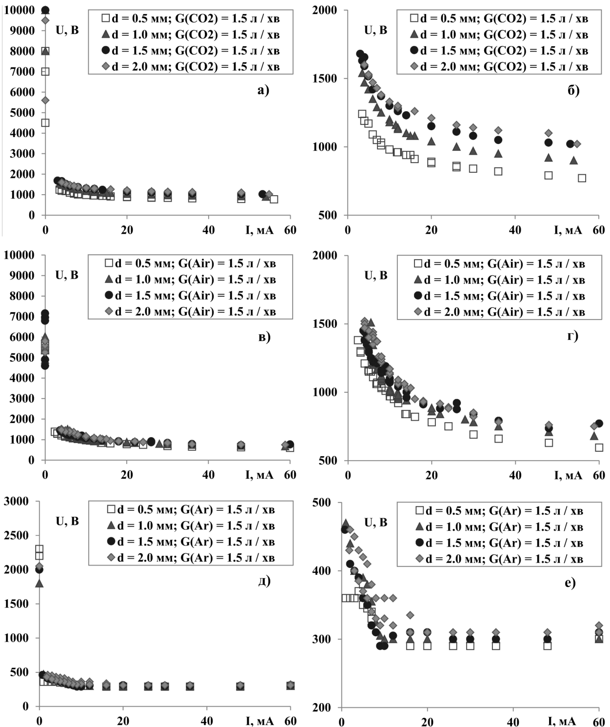
Рис. 6. Виміряні вольт-амперні характеристики в потоках G = 1,5 л/хв: CO 2 (а, б), повітря (в, г) та Ar (д, е) за використання різних d та негативній полярності високовольтного електрода
