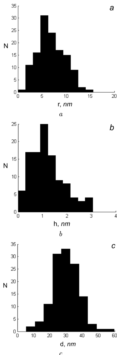
Рис. 4. Розподіли наночастинок срібла за радіусами (а), висотами (b) та відстанню між ними (c), визначені з АСМ-зображень плівки срібла d_m = 1,0 нм, напильної на позитивно заряджену поверхню LiNbO 3
