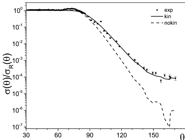
Рис. 5. Експериментальні дані по пружному розсіяню ^{16}\text{O} + ^{208}\text{Pb} для енергії пучка 95 MeV (Exp) [40] і розрахунки в рамках оптичної моделі з використанням ядерно-ядерного потенціалу як з урахуванням (kin), так і без урахування внеску кінетичної енергії (nokin)
