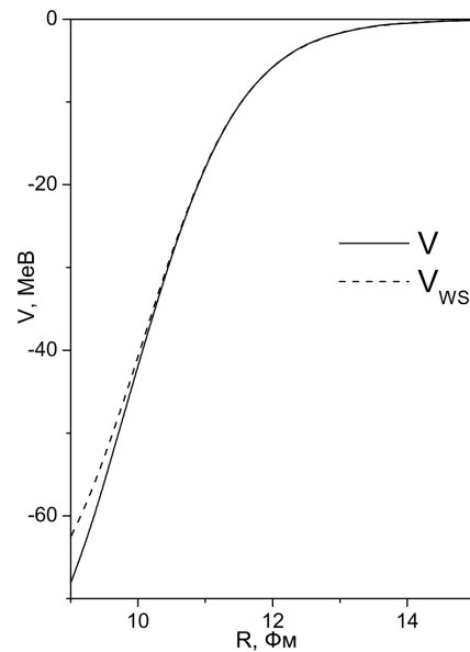
Рис. 3. Апроксимація ядерної частини одержаного потенціалу ядерно-ядерної взаємодії без урахування внеску кінетичної енергії нуклонів за допомогою потенціалу Вудса–Саксона в околі точки дотику \approx 10 Фм
