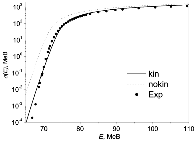
Рис. 4. Перерізи підбар'єрного злиття ^{16}\text{O} + ^{208}\text{Pb} як з урахуванням (kin), так і без урахування (nokin) внеску кінетичної енергії, а також експериментальні дані (Exp) [41]
