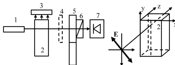
Рис. 1. Геометрія експерименту для реєстрації термопружності, індукованої радіаційним охолодженням і нагріванням: 1 – He–Ne лазер, 2 – зразок, 3 – електротермічний елемент, 4 – компенсаторна фазова пластинка, 5 – фотопружний модулятор поляризації, 6 – поляризатор, 7 – Si-фотодетектор
