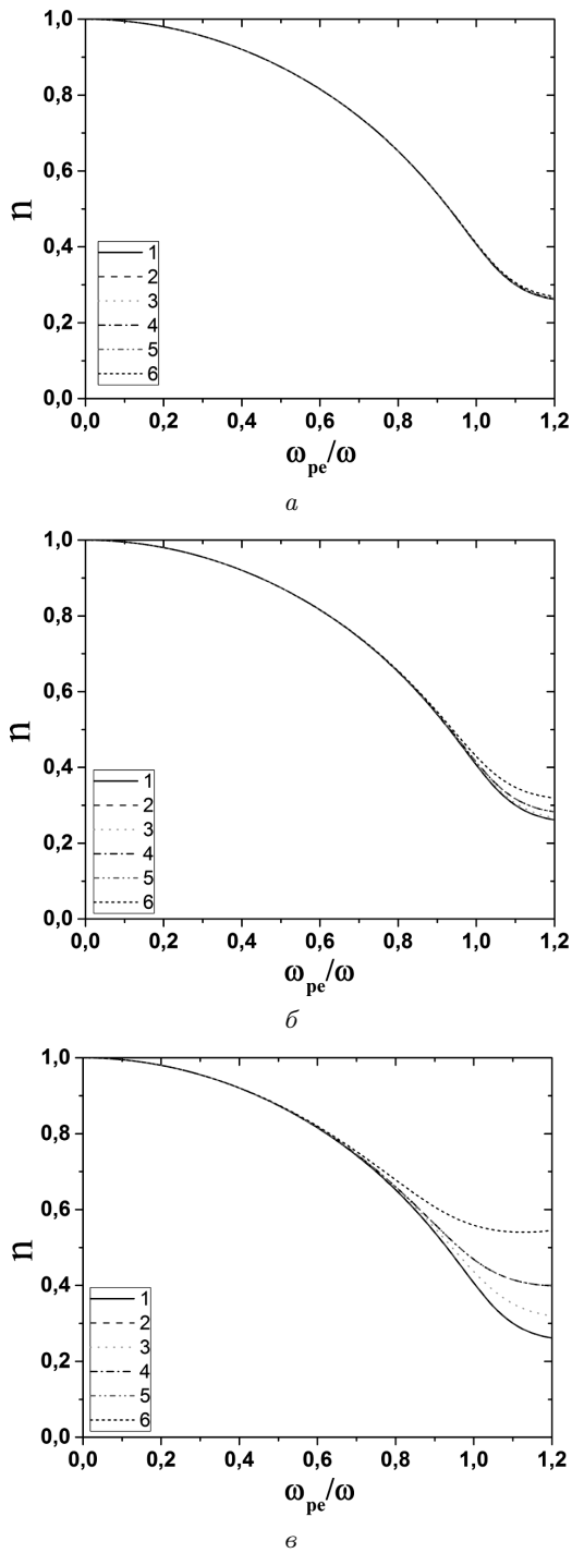
Рис. 5. Залежність показника заломлення від співвідношення \omega_{pe}/\omega для різноманітних наближень: а - N_d = 10^{10} \text{ м}^{-3} ; б - N_d = 10^{11} \text{ м}^{-3} ; в - N_d = 10^{12} \text{ м}^{-3} . 1; 2; 3; 4; 5; 6 - позначення див. у тексті ( r_d = 1 \cdot 10^{-6} \text{ м} , N_i = 1 \cdot 10^{19} \text{ м}^{-3} , N_n = 10^{24} \text{ м}^{-3} , T_e = 3000 \text{ К} , T_i = 0,1 T_e \text{ К} )
