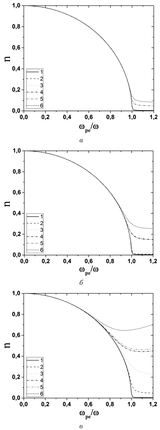
Рис. 6. Залежність показника заломлення від відношення \omega_{pe}/\omega для різноманітних наближень: а - N_d = 10^{10} \text{ м}^{-3} ; б - N_d = 10^{11} \text{ м}^{-3} ; в - N_d = 10^{12} \text{ м}^{-3} . 1; 2; 3; 4; 5; 6 - позначення див. у тексті ( r_d = 1 \cdot 10^{-6} \text{ м} , N_i = 1 \cdot 10^{16} \text{ м}^{-3} , N_n = 10^{20} \text{ м}^{-3} , T_e = 1 \text{ eВ} , T_i = 0,1 T_e \text{ eВ} )
