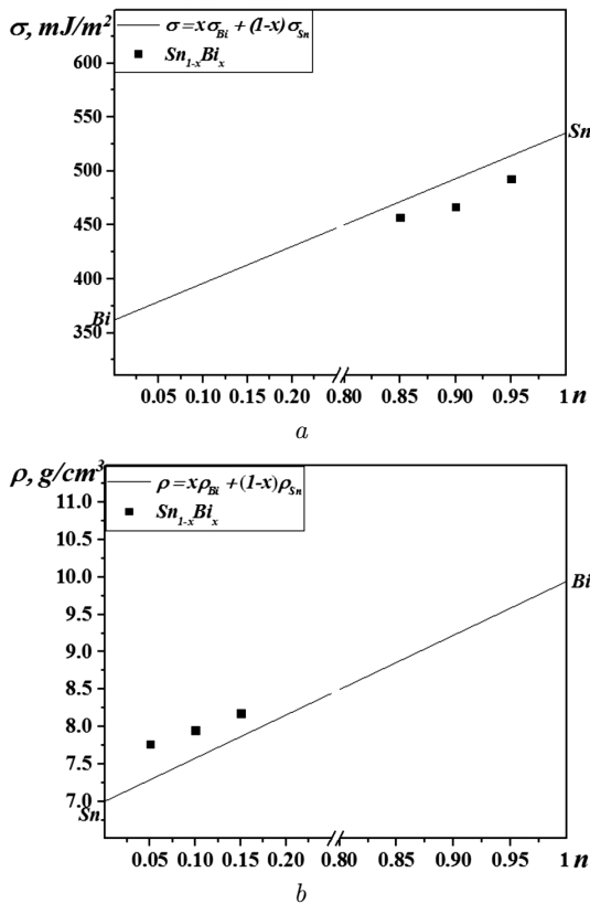
Рис. 4. Якісна інтерпретація впливу домішки Ві на КПН (а) та густину (b) рідкого олова
