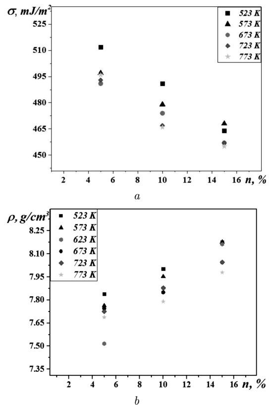
Рис. 6. Ізотерми ПН (а) та густини (b) розплавів системи Sn–Bi при різних температурах
