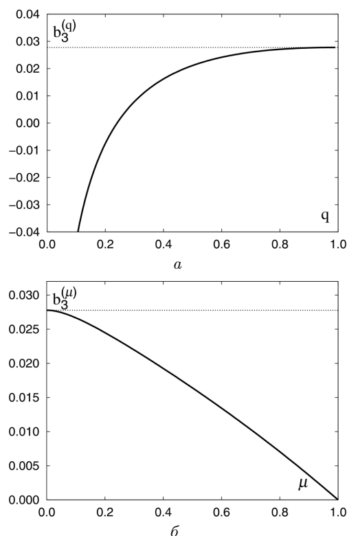
Рис. 4. Третій віріальний коефіцієнт b_3 для вимірності простору D = 2 . Графік (а) відповідає q -деформації, (б) – \mu -деформації
