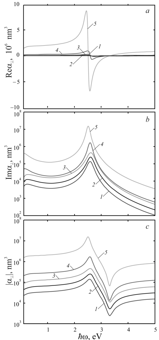
Рис. 3. Частотні залежності дійсної (а) та уявної частин (b), а також модуля (с) поперечної компоненти поляризованості стрижнеподібних частинок золота у формі витягнутого сфероїда за тих самих значень параметрів, що і на рис. 2
