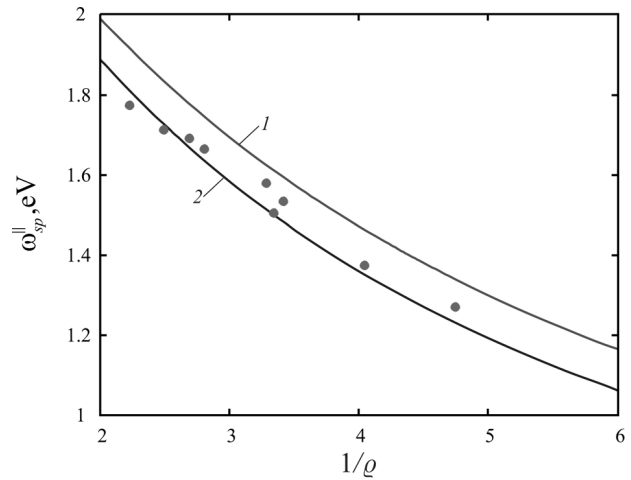
Рис. 7. Розраховані залежності частоти поздовжнього ППР від величини зворотного аспектного відношення: 1 – модель витягнутого сфероїда (розмірний параметр – аспектне відношення \varrho ); 2 – модель еквівалентного витягнутого сфероїда (розмірний параметр – ефективне аспектне відношення \varrho_{\text{eff}} ); точки – експериментальні результати з [26]
