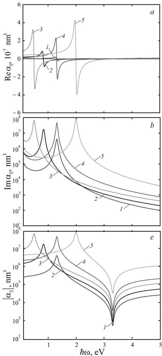
Рис. 2. Частотні залежності дійсної (а) та уявної частин (b), а також модуля (с) поздовжньої компоненти поляризованості стрижнеподібних частинок золота у формі витягнутого сфероїда: 1 – b = 10 нм, a = 50 нм; 2 – b = 10 нм, a = 100 нм; 3 – b = 10 нм, a = 200 нм; 4 – b = 20 нм, a = 100 нм; 5 – b = 50 нм, a = 100 нм
