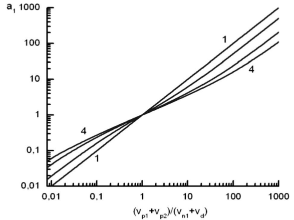
Рис. 7. Залежність параметра a_1 від співвідношення загальних концентрацій центрів (v_{p_1} + v_{p_2})/(v_{n_1} + v_d) при \delta = 1 (1), 2 (2), 5 (3), 10 (4)
