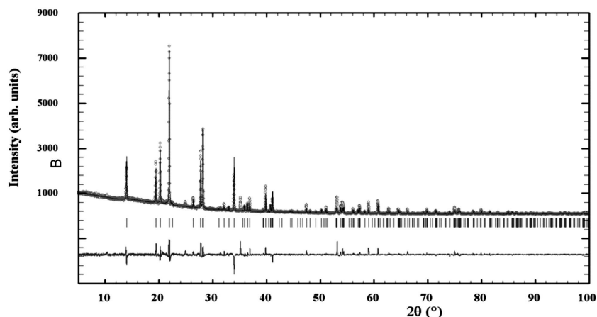
Рис. 1. Експериментальна (кільця), теоретична (суцільна лінія) та різницева (унизу) дифрактограма зразка \beta\text{-LiNH}_4\text{SO}_4 : Mn (5 wt.%)
