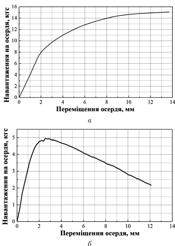
Рис. 3. Силкові характеристики магнітних пружин: базова модель (а) та пружина з магнітопроводом замість зовнішнього постійного магніту (б)
