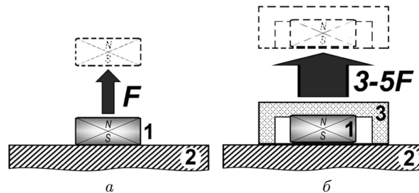
Рис. 2. Схема використання магнітопроводу для зміцнення робочої точки постійного магніту на кривій розмагнічування: постійний магніт на феромагнітній площині (а), такий самий постійний магніт і з магнітопроводом (б), постійний магніт (1), феромагнітна площина (2), магнітопровід (3)
