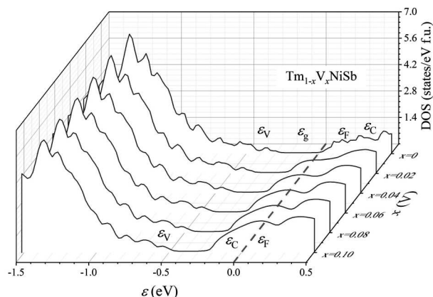
Рис. 4. Розподіл густини електронних станів у \text{Tm}_{1-x}\text{V}_x\text{NiSb} (метод KKR-CPA) для 0 \leq x \leq 0.1 . Рівень Фермі зсунуто до 0 eV
