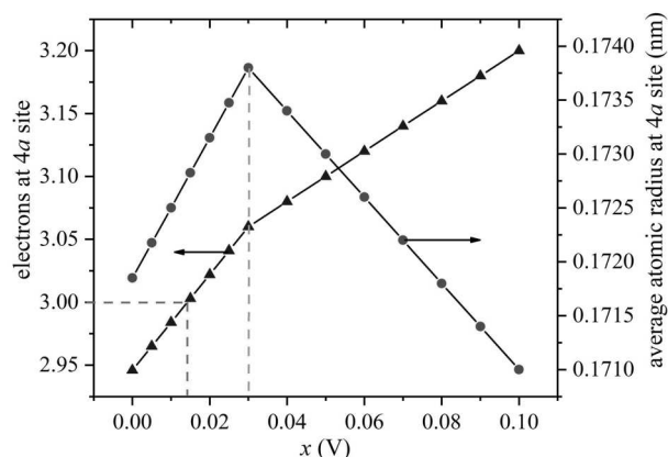
Рис. 3. Вплив одночасного заміщення атомів Тм і вакансій в позиції 4а на атоми V у неупорядкованій структурі \text{Tm}_{1-x}\text{V}_x\text{NiSb} на кількість валентних електронів, що припадають на один атом, і середній атомний радіус
