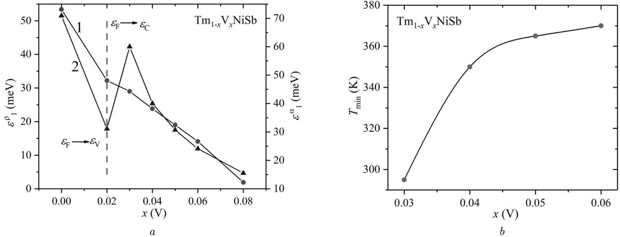
Рис. 11. Зміна значень (а) енергій активації \epsilon_1^p(x) [рівняння (1)] та \epsilon_1^\alpha(x) [рівняння (2)] та (б) температури T_{\min} , що залежать від \alpha(1/T, x) , для \text{Tm}_{1-x}\text{V}_x\text{NiSb}
