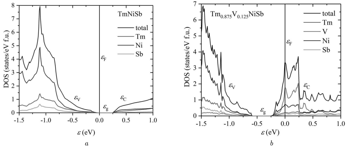
Рис. 5. Розподіл густини електронних станів у впорядкованих TmNiSb (a) і Tm_{0,875}V_{0,125}NiSb (b) (PAW метод). Рівень Фермі зсунуто до 0 eV
