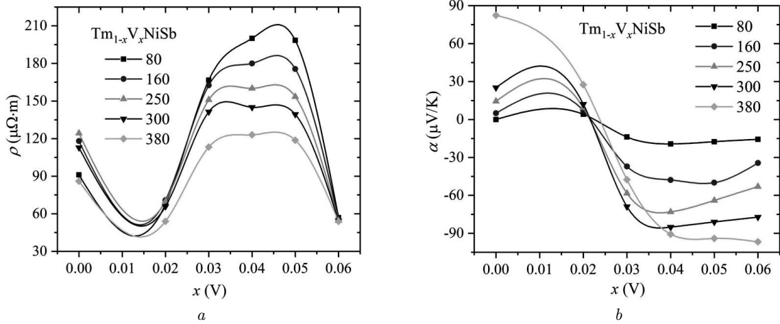
Рис. 10. Залежності (а) питомого опору \rho(x, T) і (б) коефіцієнта термо-ерс \alpha(x, T) у \text{Tm}_{1-x}\text{V}_x\text{NiSb} при різних температурах
