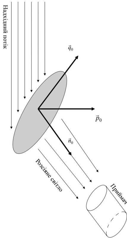
Рис. 4. Використана Петром Томчуком схема розсіювання малою сфероїдальною частинкою електромагнітної хвилі для аналізу впливу форми частинки на переріз розсіювання: вектор \mathbf{n}_0 визначає напрямок спостереження, вектор \mathbf{p}_0 задає поляризацію вихідного світлового потоку, вектор \mathbf{q}_0 задає орієнтацію осі симетрії сфероїда (репродукція рисунку з роботи [92])
