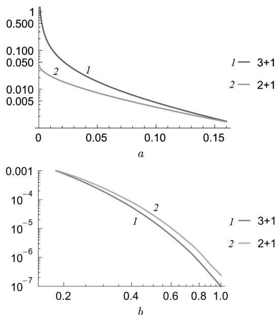
Рис. 2. Індукований вакуумний магнітний потік у безрозмірних одиницях у (2 + 1)-просторі-часі ( em^{-1}\Phi_1^{(d=2)} ) та у (3 + 1)-просторі-часі ( e\pi\Phi_1^{(d=3)} ) як функція товщини трубки mr_0 для випадків mr_0 < 0,16 (a) та mr_0 > 0,16 (b)
