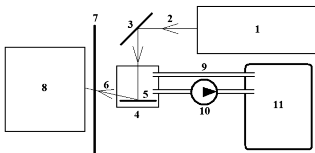
Рис. 1. Схема експериментального пристрою для дослідження сенсорних властивостей плівкових зразків до молекул ацетону в повітрі. Див. пояснення в тексті
