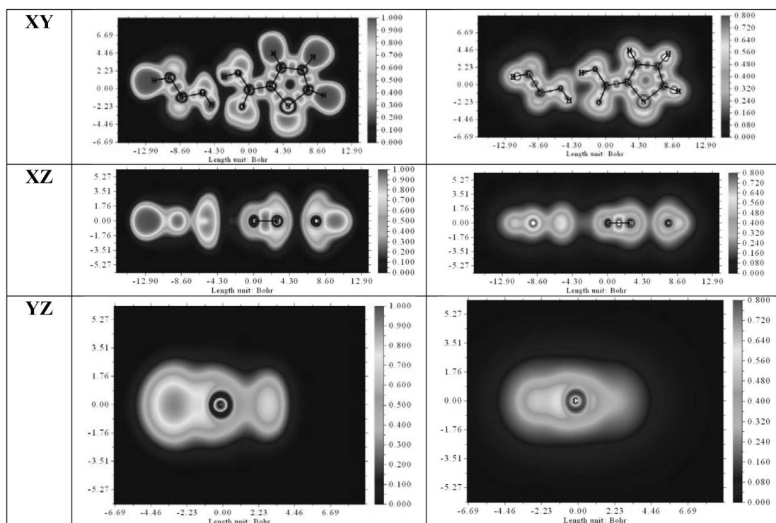
Рис. 10. ELF (ліва панель) та LOL (права панель) мапи комплексу TCA + EtOH
