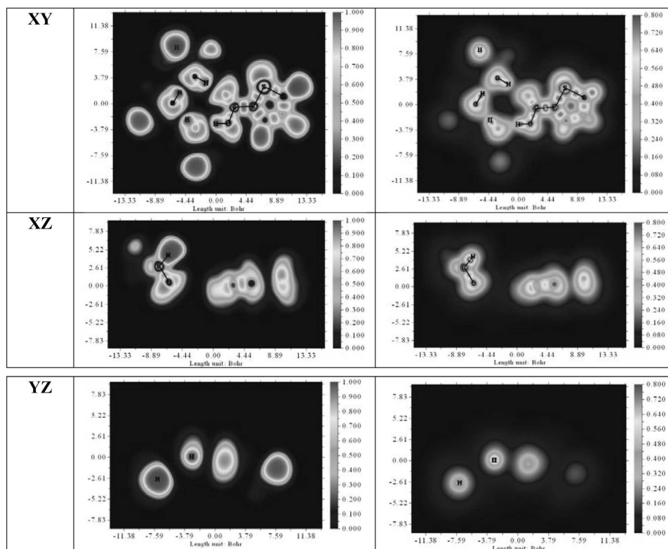
Рис. 12. ELF (ліва панель) та LOL (права панель) мапи комплексу TCA + (EtOH) 3
