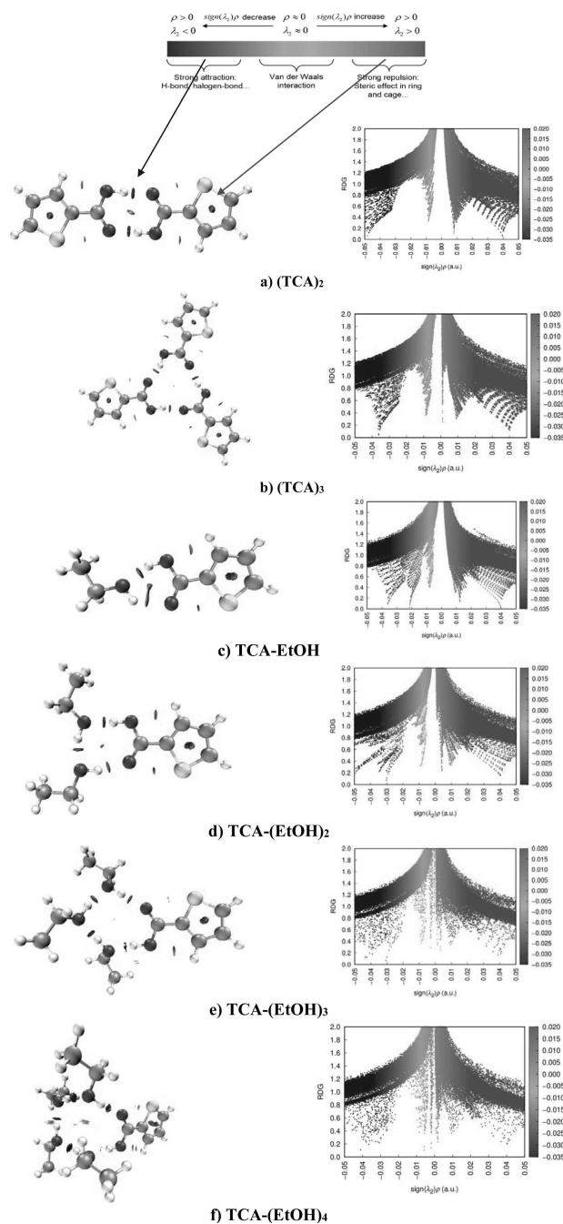
Рис. 6. NCI та RDG-аналізи (\text{TCA})_n ( n = 1-3 ) та комплексів \text{TCA} + (\text{EtOH})_m ( m = 1-4 )
