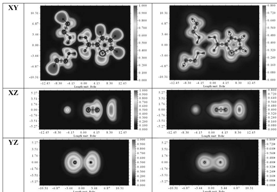
Рис. 11. ELF (ліва панель) та LOL (права панель) мапи комплексу TCA + (EtOH) 2
