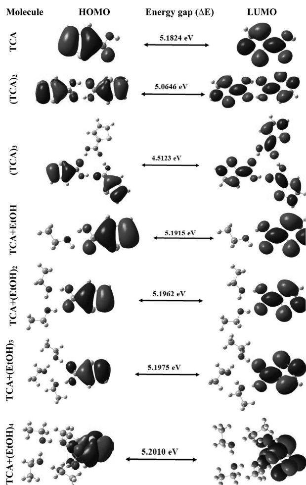
Рис. 4. FMO діаграми (TCA)_n ( n = 1-3 ) та комплексів TCA + (EtOH)_m ( m = 1-4 )
