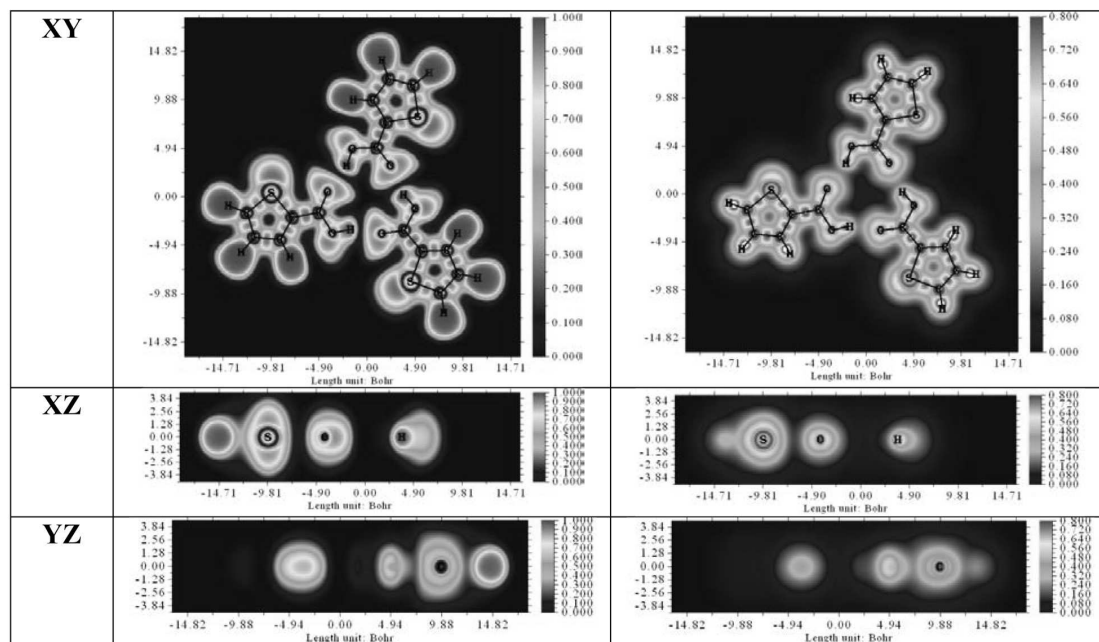
Рис. 9. ELF (ліва панель) та LOL (права панель) мапи тримеру (TCA) 2
