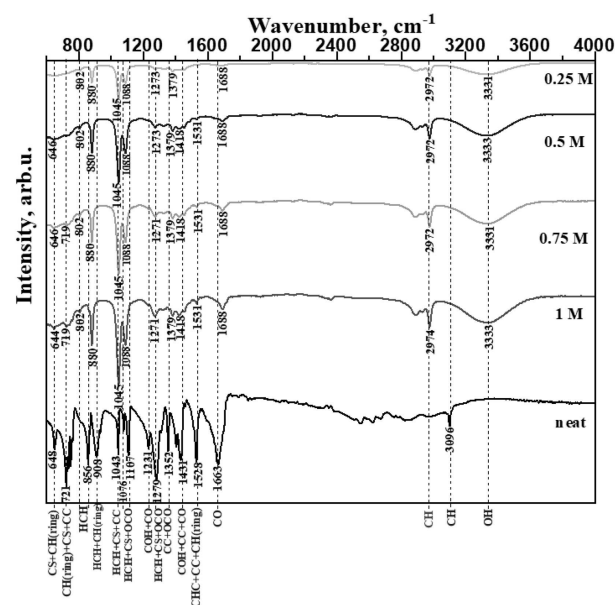
Рис. 2. ІЧ спектри ТСА в розчинах EtOH
