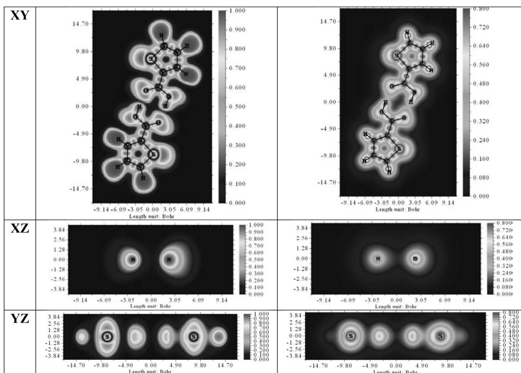
Рис. 8. ELF (ліва панель) та LOL (права панель) мапи димеру (TCA) 2
