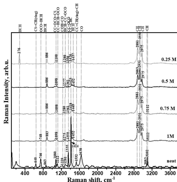
Рис. 1. Спектри комбінаційного розсіювання ТСА в розчинах EtOH
