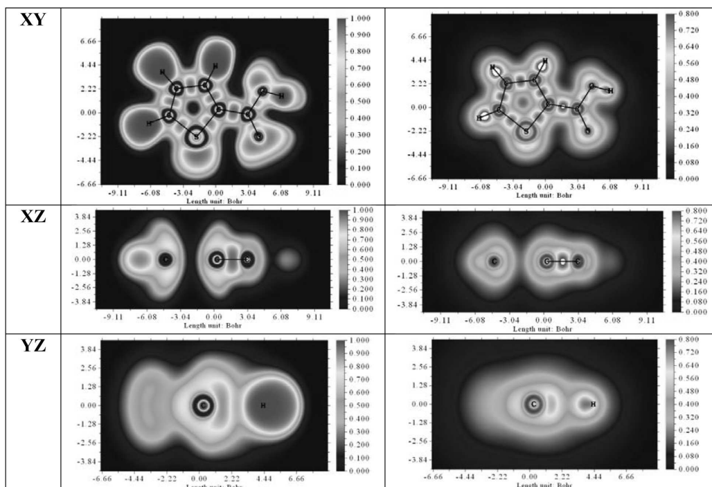
Рис. 7. ELF (ліва панель) та LOL (права панель) мапи молекули TCA
