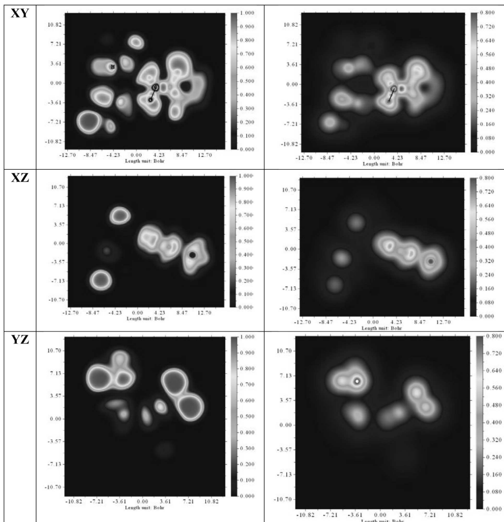
Рис. 13. ELF (ліва панель) та LOL (права панель) мапи комплексу TCA + (EtOH) 4
