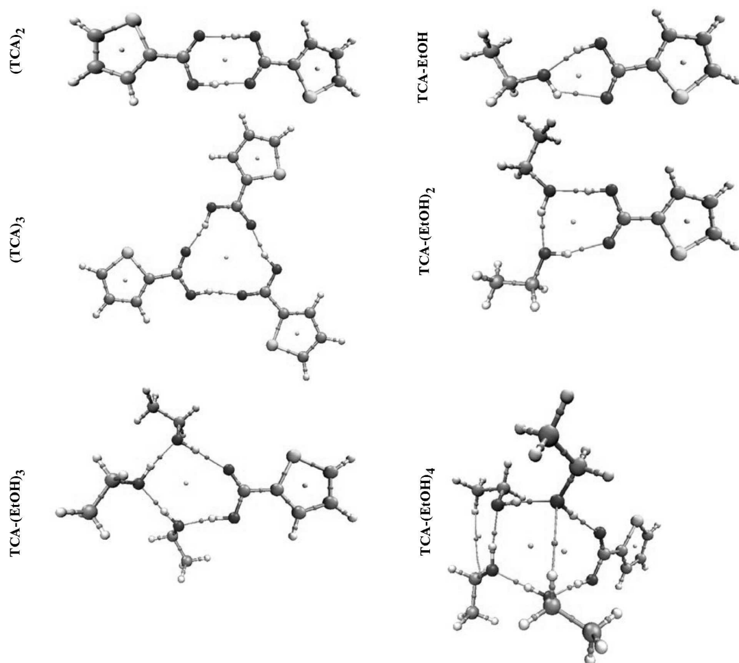
Рис. 5. AIM аналіз (TCA)_n ( n = 1-3 ) та комплексів TCA + (EtOH)_m ( m = 1-4 )
