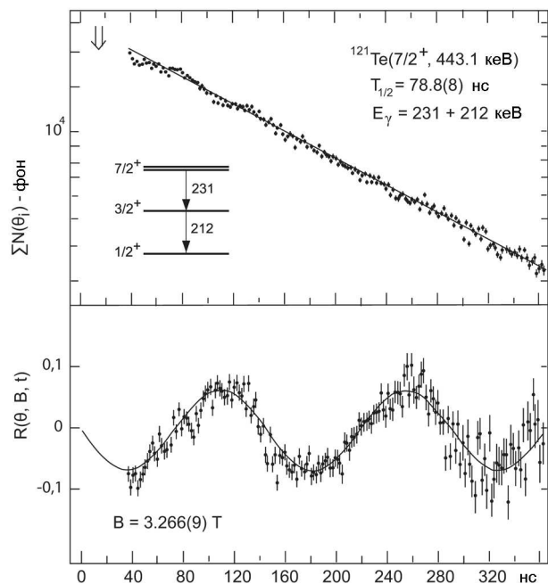
Рис. 3. Сума часових спектрів, скоригована на фон (див. текст) (а), та часово-диференціальна спінова прецесія R(t) для переходів 212 та 231 кеВ, що дезбуджують стан 7/2^+ в ^{121}\text{Te} (б). Суцільні криві є результатом достосування згідно з рівнянням (3)
