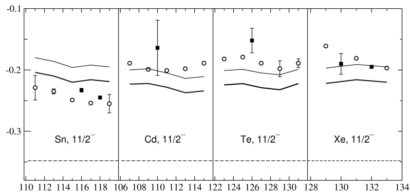
Рис. 5. g -фактори станів 11/2^- та 10^+ в ізотопах ядер Sn, Cd, Te та Xe. Штрихові лінії – одночастинкові значення g_{SP} , тонкі суцільні лінії – значення g_T^{ef1} , жирні суцільні лінії – значення g_T^{ef2} , білі кола – експериментальні g -фактори 11/2^- станів, чорні квадрати – g -фактори 10^+ станів
