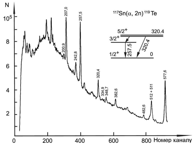
Рис. 2. \gamma -спектр реакції ^{117}Sn(\alpha, 2n)^{119}Te на товстій ізотопній мішені з олова
