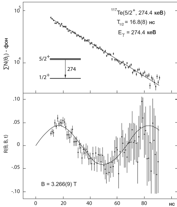
Рис. 1. Сума часових спектрів, скоригована на фон (див. текст) (а), та часово-диференціальна спінова прецесія R(t) для переходу 274 кеВ, що дезбуджує стан 5/2^+ в ^{117}\text{Te} (б). Суцільні криві є результатом достосування згідно з рівнянням (3)
