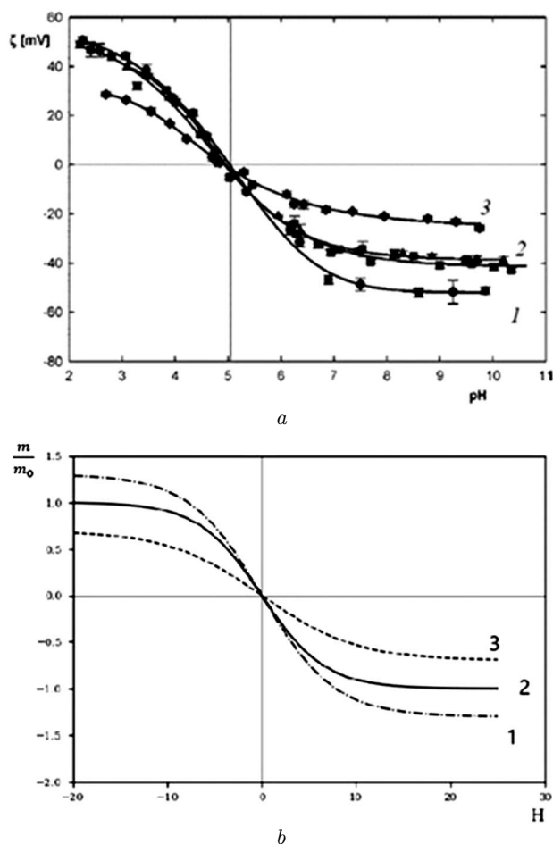
Рис. 1. Експериментальна залежність дзета-потенціалу альбуміну ( \zeta_{\text{alb}} ) від показника рН [9] (а) та схематична залежність відносної намагніченості різних парамагнетиків m/m_0 від значення напруженості зовнішнього магнітного поля H (б). Криві на рис. 1, а відповідають різним чисельним густинам солі хлориду натрію: n_s^{(1)} = 0,6 \cdot 10^{18} \text{ см}^{-3} (1), n_s^{(2)} = 1,8 \cdot 10^{18} \text{ см}^{-3} (2), n_s^{(3)} = 6 \cdot 10^{18} \text{ см}^{-3} (3). Криві на рис. 1, б відповідають різним температурам парамагнетика: крива 1 відповідає найнижчій температурі, крива 3 – найвищій
