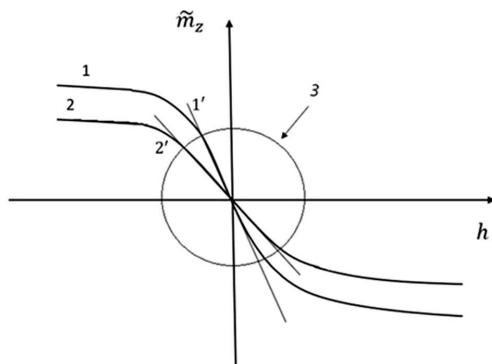
Рис. 6. Схематичні криві залежності намагніченості парамагнетика m_z як функція напруженості зовнішнього магнітного поля h . Цифрами 1 та 2 позначені криві залежності за різних температур, прямі 1' та 2' – це дотичні до вказаних кривих в околі критичної точки, який на рисунку обмежений колом. Область застосування теорії Ландау обмежена кривою 3
