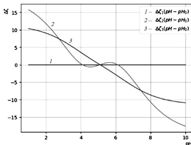
Рис. 8. Значення \Delta \zeta_{\text{alb}}(x) , які відповідають кривим, зображеним на рис. 1
