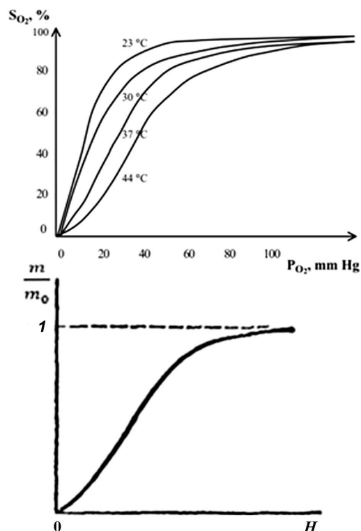
Рис. 9. Залежність ступеня насиченості гемоглобіну киснем в крові ( SO_2 ) як функція парціального тиску кисня в альвеолах ( PO_2 ) [21] (а) та схематична залежність намагніченості парамагнетика m/m_0 від значення напруженості зовнішнього магнітного поля H (б)
