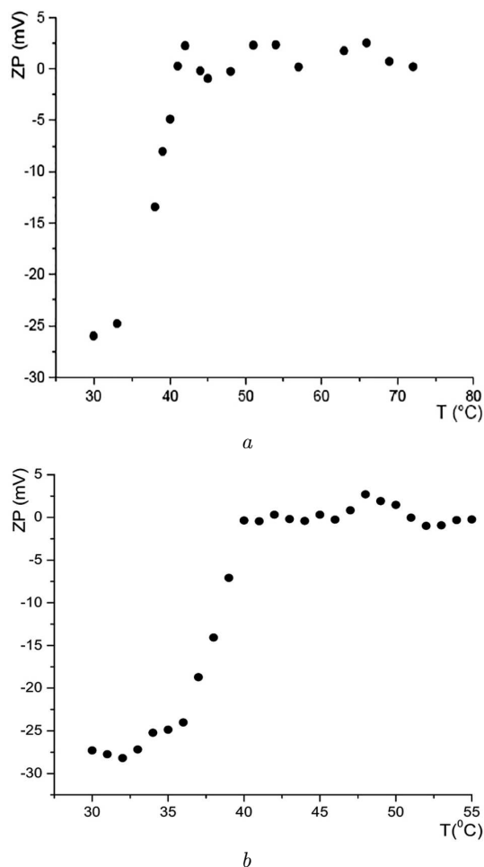
Рис. 3. Температурна залежність дзета-потенціалу для водно-сольових розчинів альбуміну (а) та фібриногену (б) при рН = 7,4 і концентрації хлориду натрію 0,075 моль/л [15]
