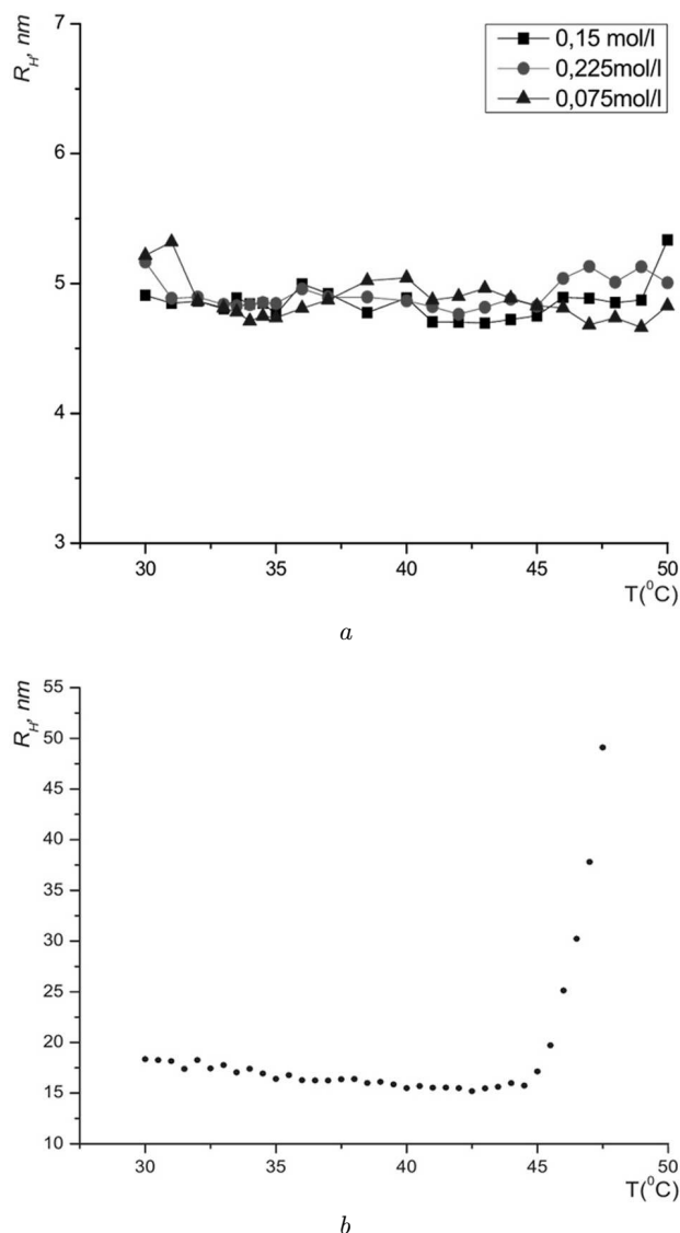
Рис. 4. Температурна залежність гідродинамічного радіуса альбуміну (а) та фібриногену (b) [15, 16]
