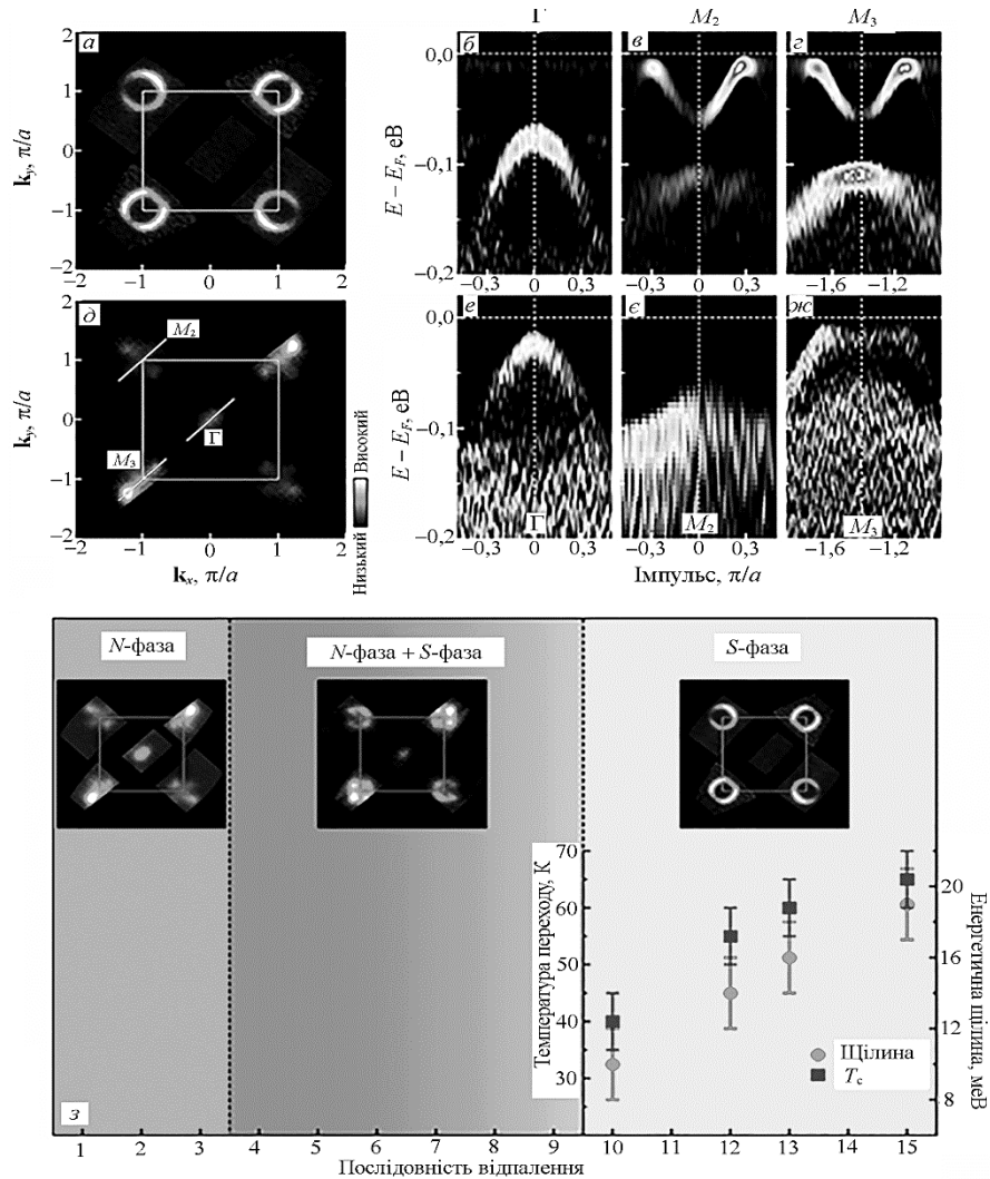
Рис. 14. Електронна структура S -фази, N -фази та фазова діаграма моношару \text{FeSe}/\text{SiTiO}_3 після відпалення у вакуумі. (а) Фермі-поверхня S -фази моношару \text{FeSe}/\text{SiTiO}_3 . (б-г) Зонна структура S -фази біля \Gamma -, M_2 - та M_3 -перерізів відповідно. (д) Фермі-поверхня N -фази моношару \text{FeSe}/\text{SiTiO}_3 . (е-ж) Зонна структура S -фази біля \Gamma - M_2 - та M_3 -перерізів, відповідно. Зонна структура на (б-г) і (е-ж) — друга похідна по енергії від оригінальної зонної структури. (з) Схематична фазова діаграма моношару \text{FeSe} -плівки в процесі відпалення. Вставки демонструють поверхню Фермі на кожній стадії процесу відпалення [35]. 14
