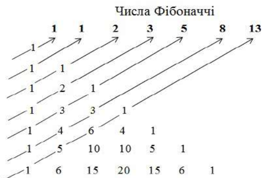
Рис. 1. Арифметичний трикутник і числа Фібоначчі
