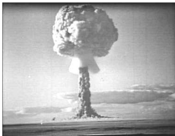
Fig. 6. RDS-1 test
