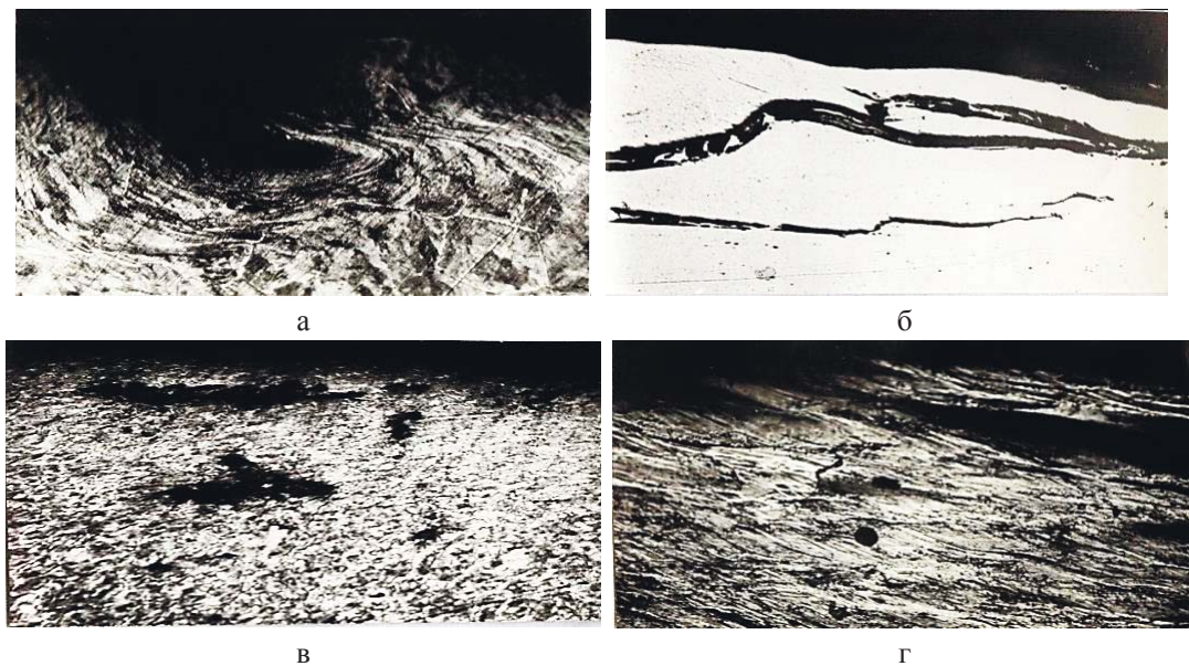
Рис. 2. Частицы износа вблизи поверхности катания в зоне интенсивной пластической деформации; а –х100, б – г –х200
