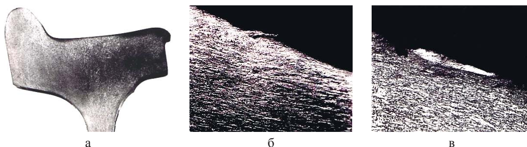
Рис. 1. Макроструктура колеса с изношенным ободом (а) и зоны структурных изменений вблизи поверхности катания (б, в – х 200)
