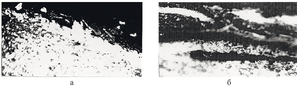
Рис. 3. Частицы износа (а) и выкрашивание «белого слоя» (б); \times 1000
