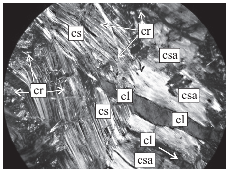
Рис. 7. Серпентиніт хризотилівий. Зб. 100. Нік. +: cs — хризотил; cl — хлорит; csa — хризотил-азбест; cr — карбонат
