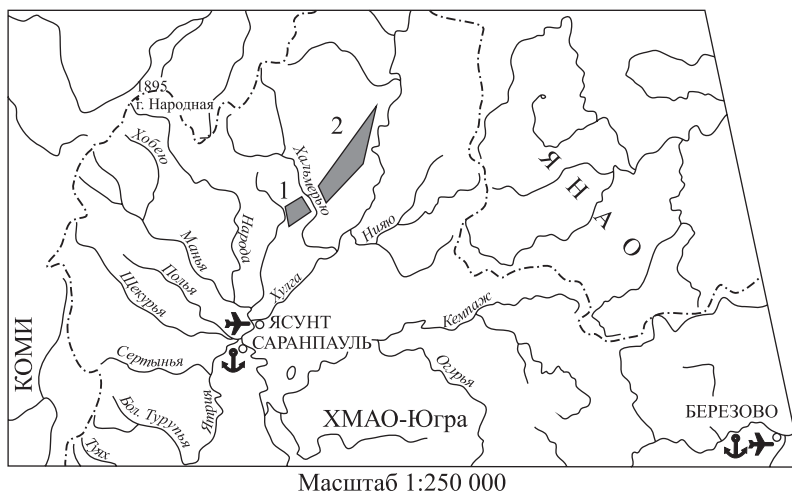
Рис. 1. Схема розміщення Сінтовожського (1) та Оліся-Мусюрського (2) масивів: ЯНАО — Ямало-Ненецький автономний округ; ХМАО-Югра — Ханті-Мансійський автономний округ Югра
