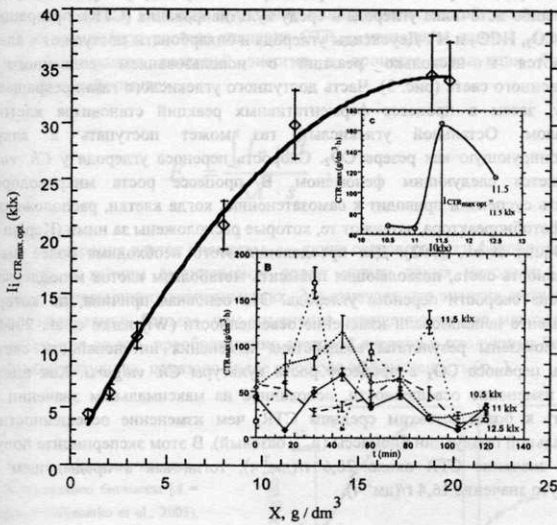
Рис. 2. Соотношение интенсивности света, максимального значения CTR ( I_{CTR_{max,opt}} ) и продукции биомассы культуры Chlorella vulgaris Beijer. (X); учтены усредненные данные, полученные из трех повторностей эксперимента.
