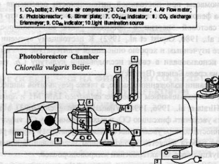
Рис. 1. Экспериментальный аппарат. 1 – CO 2 дюз; 2 – портативный компрессор; 3 – измеритель потока CO 2 ; 4 – измеритель потока воздуха; 5 – фотобиореактор; 6 – тарелка Стиррера; 7 – CO 2 out внешний индикатор; 8 – CO 2 чашка Эйренмейера; 9 – CO 2 in внутренний индикатор; 10 – источник освещения.
