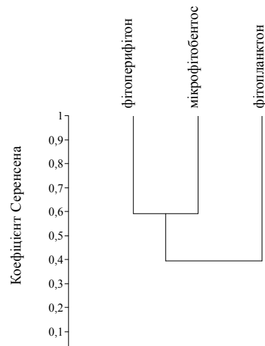
Рис. 2. Дендрограма подібності фітопланктону, мікрофітобентосу та фітоперифітону р. Західний Буг та її допливів за коефіцієнтом Серенсена в меженний період «біологічного літа» – «біологічної осені» 2018 р.
