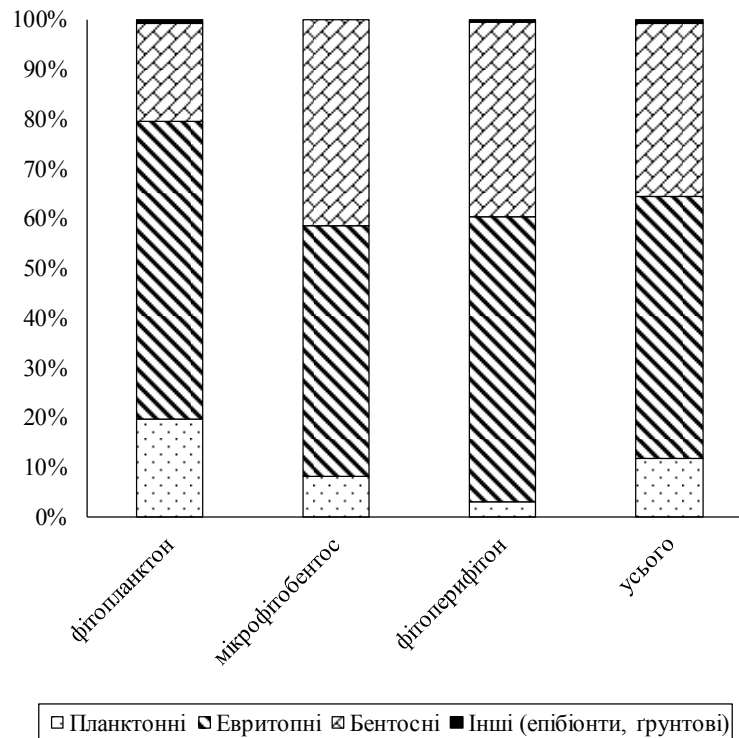
Рис. 4. Співвідношення водоростей з різною біотопічною приуроченістю (%) у фітопланктоні, мікрофітобентосі, фітоперіфітоні та альгофлорі в цілому в р. Західний Буг та її допливів у літньо-осінню межень 2018 р.
