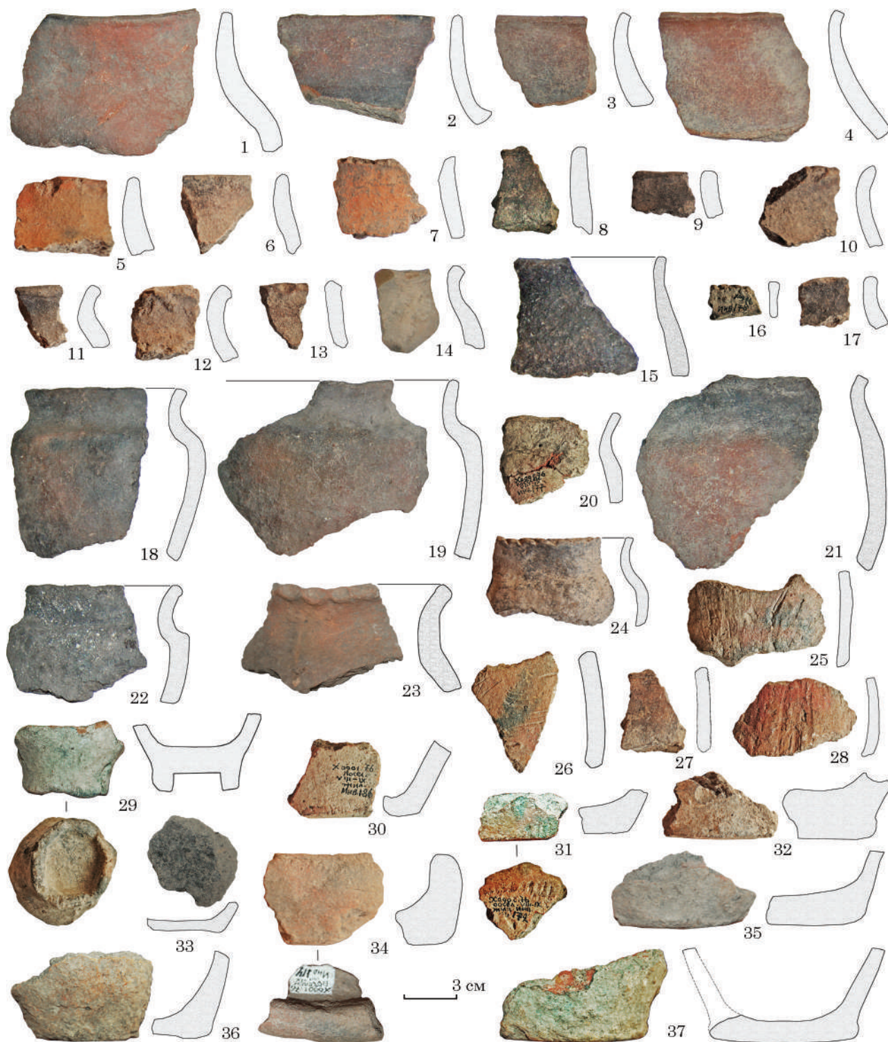
Рис. 6. Фрагменти посуду з заповнення споруди 1976 р. з Ходосівки
