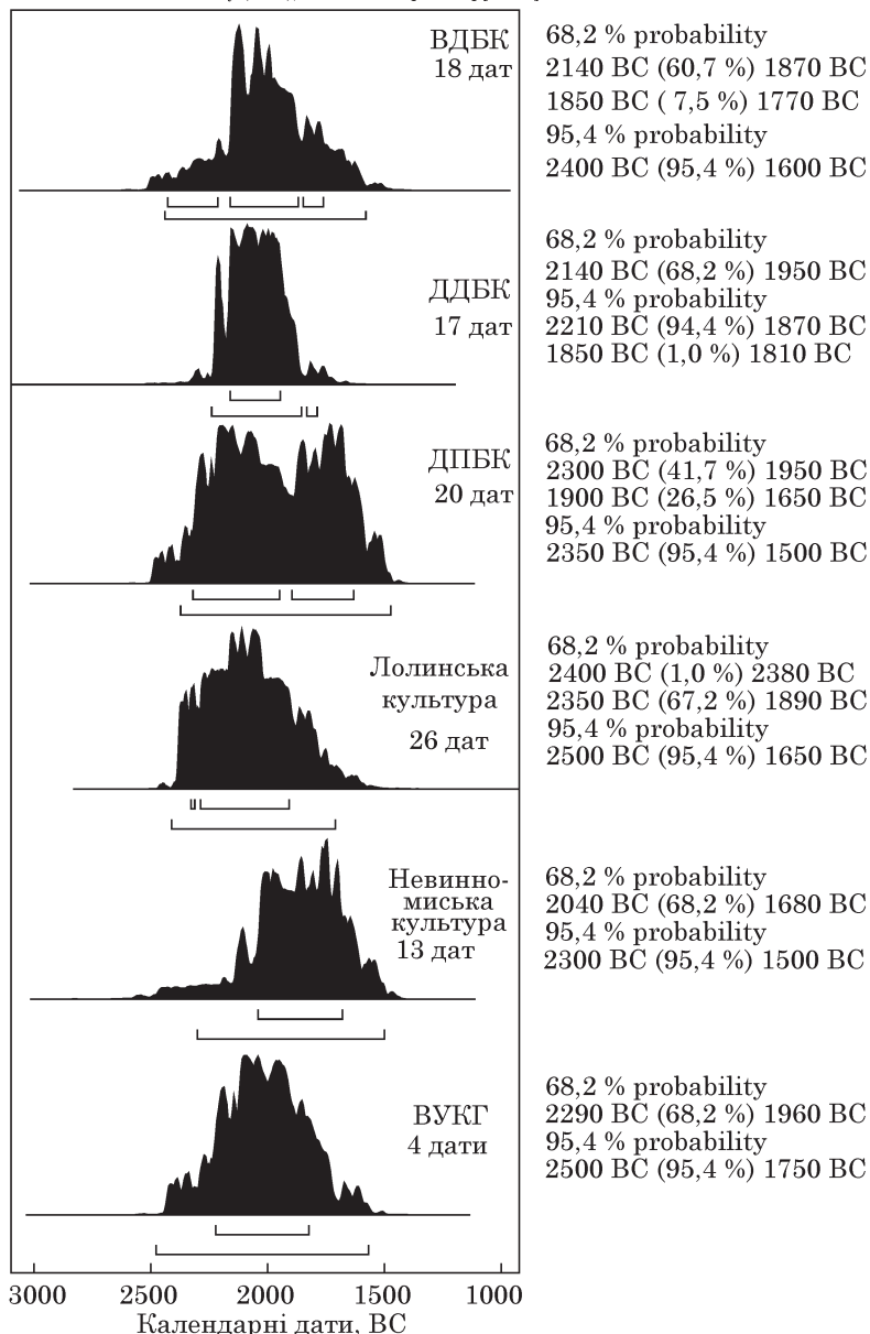
Рис. 16. Результати підсумовування (sum_probability) 14 C даних посткатакомбних культурних утворень
