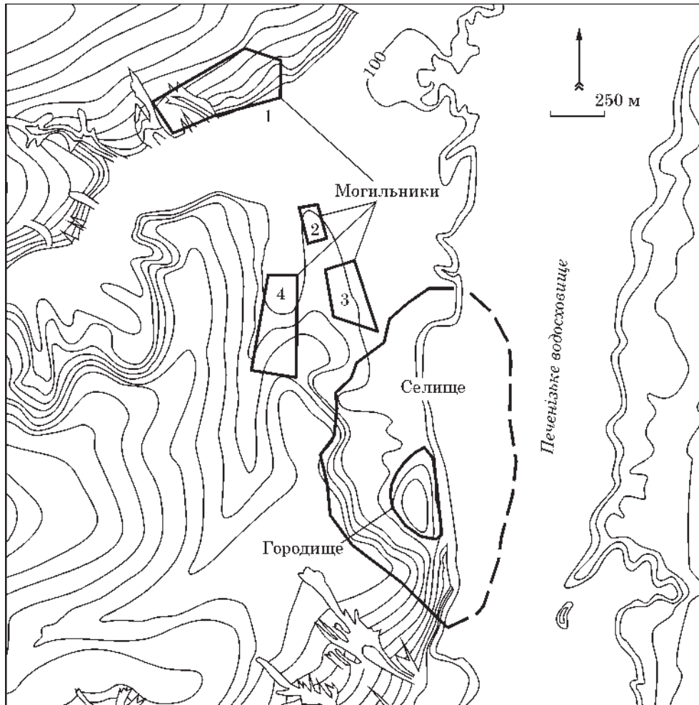
Рис. 1. План Верхньосалтівського археологічного комплексу
