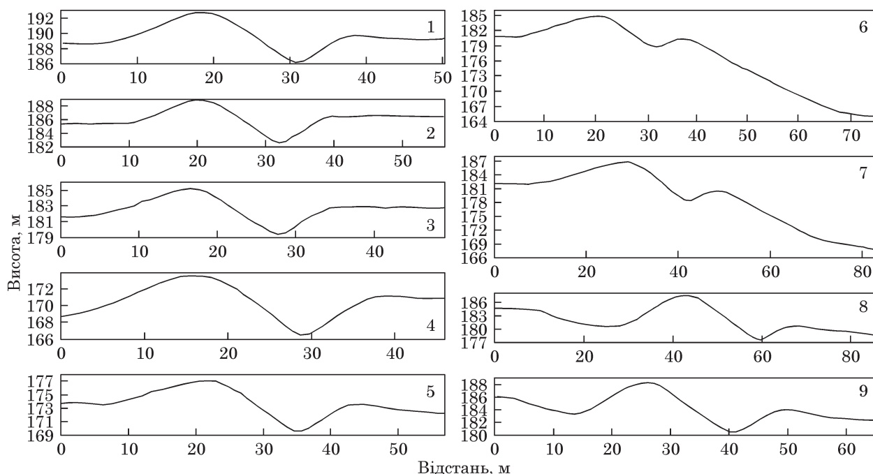
Рис. 12. Профілі валу та рову Східного укріплення (за О. Коротею; див. рис. 8)
