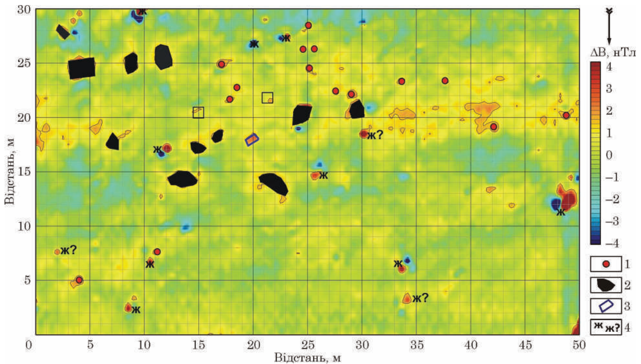
Рис. 3. Могилище Івківці. Результати геомагнітної зйомки: 1 — імовірні кремаційні поховання; 2 — імовірні скіфські житла; 3 — імовірне інгумаційне поховання; 4 — залізне сміття, сумнівні аномалії (виконала К. Бондар)
