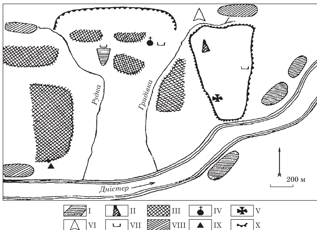
Рис. 13. План Бакоти ХІІ–ХІV ст. (за І. Винокуром і П. Горішнім): І — дитинець; ІІ — городище-замок; ІІІ — посад; ІV — церква; V — скельний печерський монастир; VI — палацова будівля; VII — кладовище; VIII — селище; IX — місце групового поховання; X — скельні урвища
