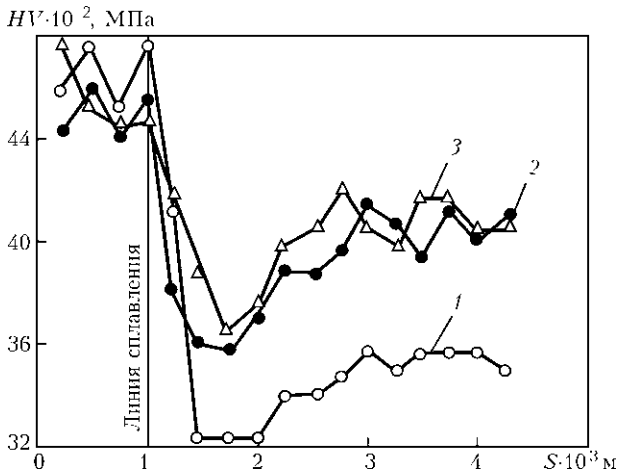
Рис. 6. Влияние погонной энергии на микротвердость HV наплавленного металла: 1 — q_3/v = 3,6 ; 2 — 2,7; 3 — 1,8 МДж/м; S — ширина ЗТВ
