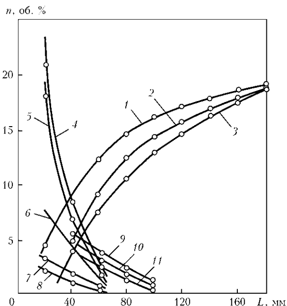
Рис. 5. Влияние исходного состава газовой смеси на содержание характерных компонентов в плазме — O_2 (1, 2, 3), [H] (4, 5, 6), H_2 (7, 8), CO (9, 10, 11) в продольном сечении струи плазмы: 1 — \alpha = 1,00 ; 2 — 0,84; 3 — 0,63; 4 — 0,63; 5 — 0,84; 6 — 1,00; 7 — 0,84; 8 — 0,63; 9 — 1,00; 10 — 0,84; 11 — 0,63
