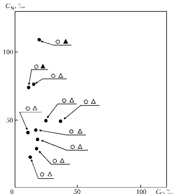
Рис. 10. Влияние газов на пористость металла швов (условия: углеродистая сталь, горизонтальное положение, сварка с проплавлением): ●, ○ — соответственно наличие и отсутствие пористости для пластин толщиной 100 мм; ▲, △ — 150
