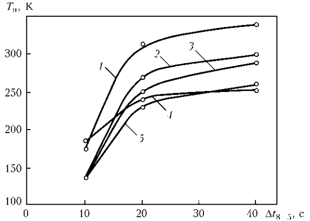
Рис. 14. Влияние расчетного времени охлаждения \Delta t_{8/5} на температуру перехода к разрушению металла шва T_{10} (условия: сталь SQV 2B, расположение — 1/2b ; положение надреза — металл шва): 1 — непосредственно после сварки; 2–5 — параметры отпуска соответственно 17,7 (2); 18,2 (3); 18,8 (4); 19,7 (6)
