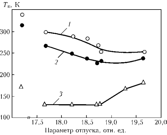
Рис. 13. Влияние параметра отпуска на температуру перехода к разрушению металла шва T_{10} (условия: сталь SQV2B, расположение — 1/2b ; положение надреза — металл шва; 1, 2 — b = 120 мм соответственно высокое и нормальное тепловложение; 3 — b = 20 мм)
