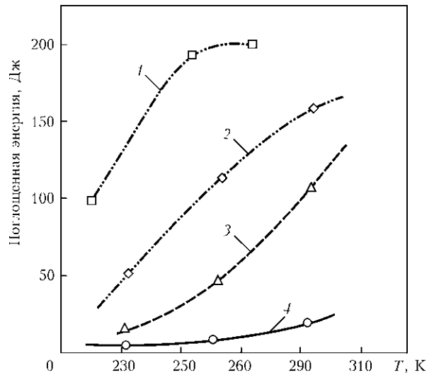
Рис. 12. Энергия, поглощенная при испытании образцов по Шарпи стали SQV 2В (условия: b = 90 мм; расположение — 1/2b ; ТОПС — 888 К; 14,4 кс): 1 — металл ЗТВ; 2 — основной металл; 3 — соединение; 4 — металл шва
