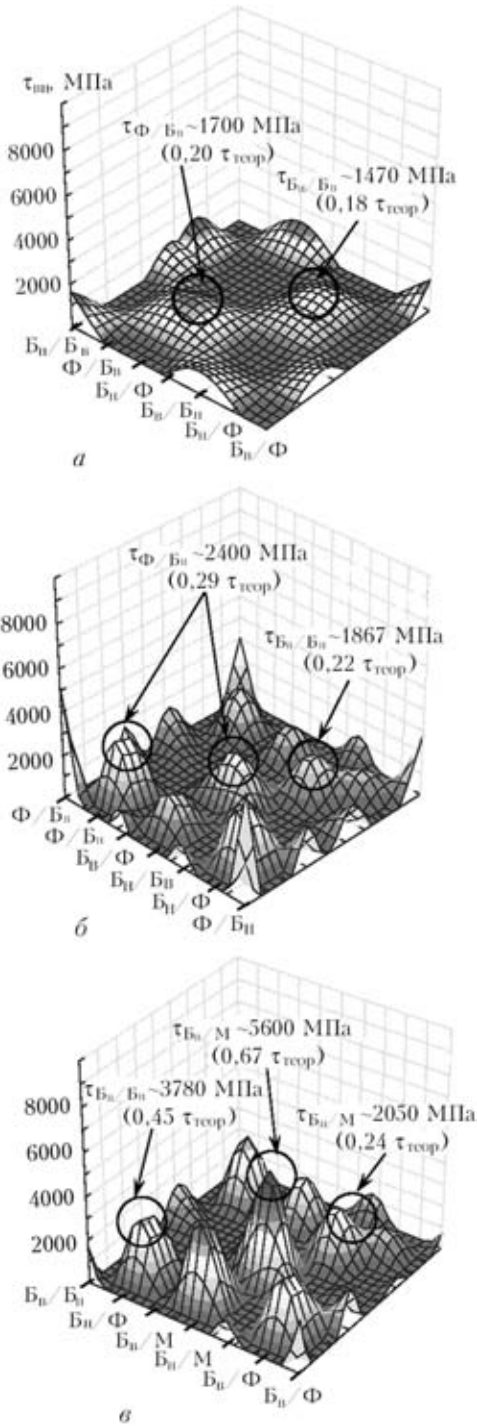
Рис. 8. Расчетные значения внутренних напряжений \tau_{вн} и теоретической прочности \tau_{теор} в различных структурных зонах их локализации ( B_n , B_v , \Phi , M и границ их сопряжений) (I зона ЗТВ) сварных соединений стали 17Х2М, полученных с использованием проволоки Св-08Х20Н9Г7Т (шов Ф-П типа) (а), Св-08Г2С (шов А-Ф типа) (б) и Св-10ХН2ГСМФТЮ (шов Б-М типа) (в)
