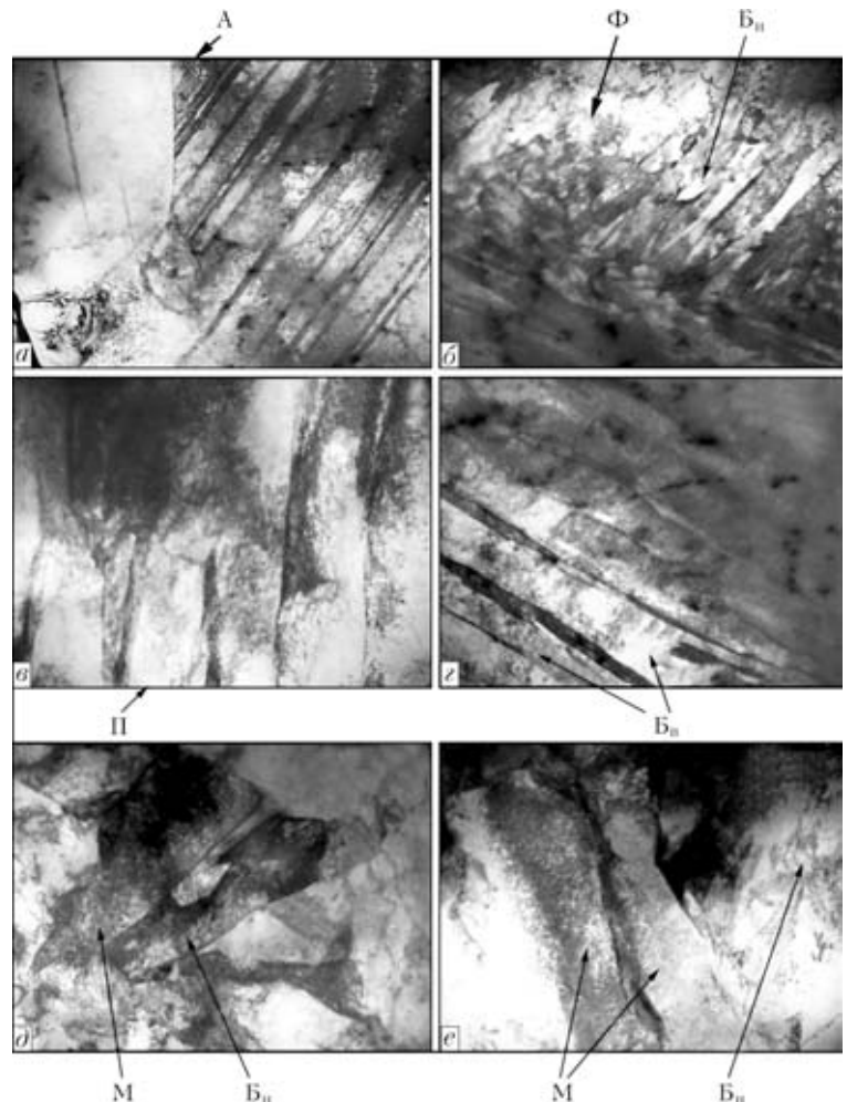
Рис. 4. Тонкая структура металла швов (а, в, д) и участков крупного зерна (I зона ЗТВ) сварных соединений стали 17X2M (б, г, е), полученных с использованием сварочных проволок Св-08Х20Н9Г7Т (а, б), Св-08Г2С (в, г), Св-10ХН2ГСМФТЮ (д, е) (а, ×10000; б, в, д, е, ×15000; г, ×20000)
