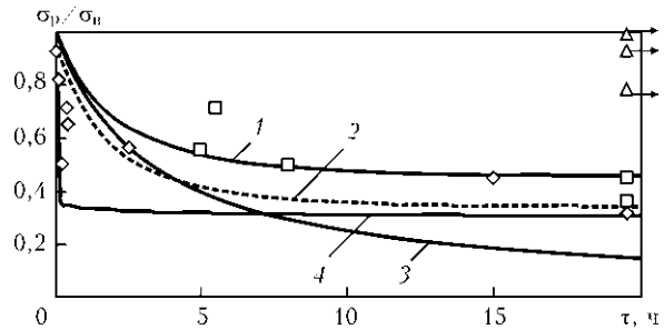
Рис. 2. Расчетные (кривые 1–4) и экспериментальные данные (значки) с разными ядрами последействия: 1, 2 — ядро последействия тела Кельвина при соответственно содержании в образце [H]_0 = 5,0 и 15 \text{ мл}/100 \text{ г} ; 3 — ядро Максвелла при [H]_0 = 5,0 \text{ мл}/100 \text{ г} ; 4 — степенное ядро при [H]_0 = 15 \text{ мл}/100 \text{ г}
