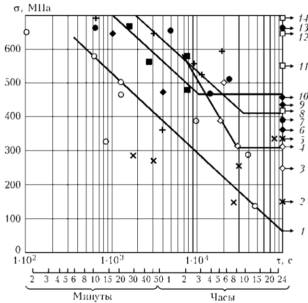
Рис. 1. Экспериментальные данные о влиянии диффузионного водорода [H]_{\text{диф}} на склонность образцов-вставок к замедленному разрушению сталей 14X2ГМР (1, 3, 4, 6, 7, 9, 11, 12, 14) и Т-1 (2, 5, 8, 10, 13): 1 — [H]_{\text{диф}} = 14,8 \text{ см}^3/100 \text{ г} ( T_{\text{ср}} = -40 \text{ }^\circ\text{C} ); 2 — [H]_{\text{диф}} = 15,0 \text{ см}^3/100 \text{ г} ( T_{\text{ср}} = -25 \text{ }^\circ\text{C} ); 3, 4 — [H]_{\text{диф}} = 5,0 \text{ см}^3/100 \text{ г} ( T_{\text{ср}} = -40 \text{ }^\circ\text{C} ); 5 — [H]_{\text{диф}} = 7,9 \text{ см}^3/100 \text{ г} ( T_{\text{ср}} = 20 \text{ }^\circ\text{C} ); 6, 9 — [H]_{\text{диф}} = 5,0 \text{ см}^3/100 \text{ г} ( T_{\text{ср}} = 20 \text{ }^\circ\text{C} ); 7 — [H]_{\text{диф}} = 7,9 \text{ см}^3/100 \text{ г} ( T_{\text{ср}} = 20 \text{ }^\circ\text{C} ); 8, 10 — [H]_{\text{диф}} = 5,0 \text{ см}^3/100 \text{ г} ( T_{\text{ср}} = 20 \text{ }^\circ\text{C} ); 11, 12, 14 — [H]_{\text{диф}} = 0,6 \text{ см}^3/100 \text{ г} ( T_{\text{ср}} = -40 \text{ }^\circ\text{C} ); 13 — [H]_{\text{диф}} = 0,6 \text{ см}^3/100 \text{ г} ( T_{\text{ср}} = 20 \text{ }^\circ\text{C} )
