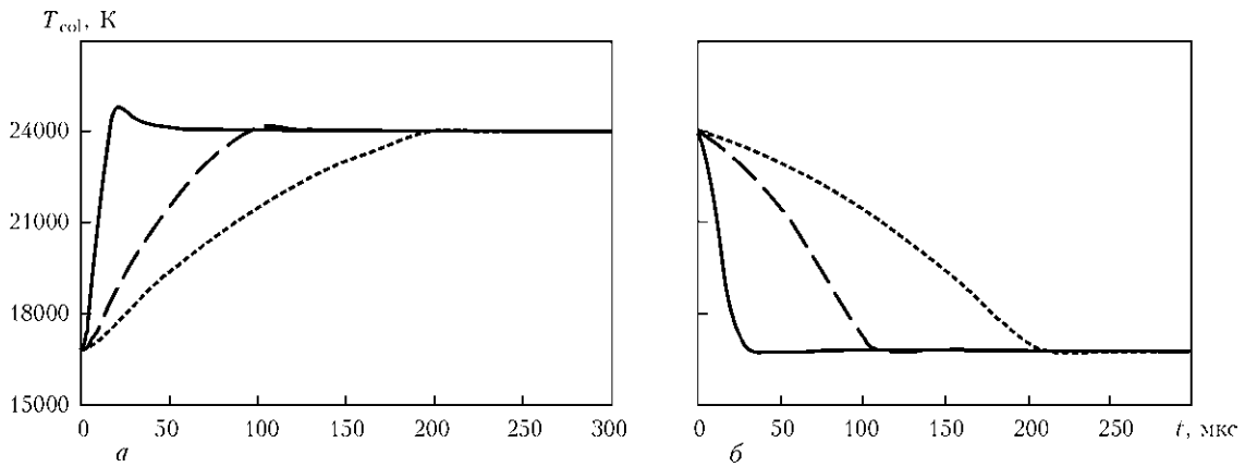
Рис. 5. Изменение температуры плазмы в центре столба дуги на переднем (а) и заднем (б) фронтах импульса тока
