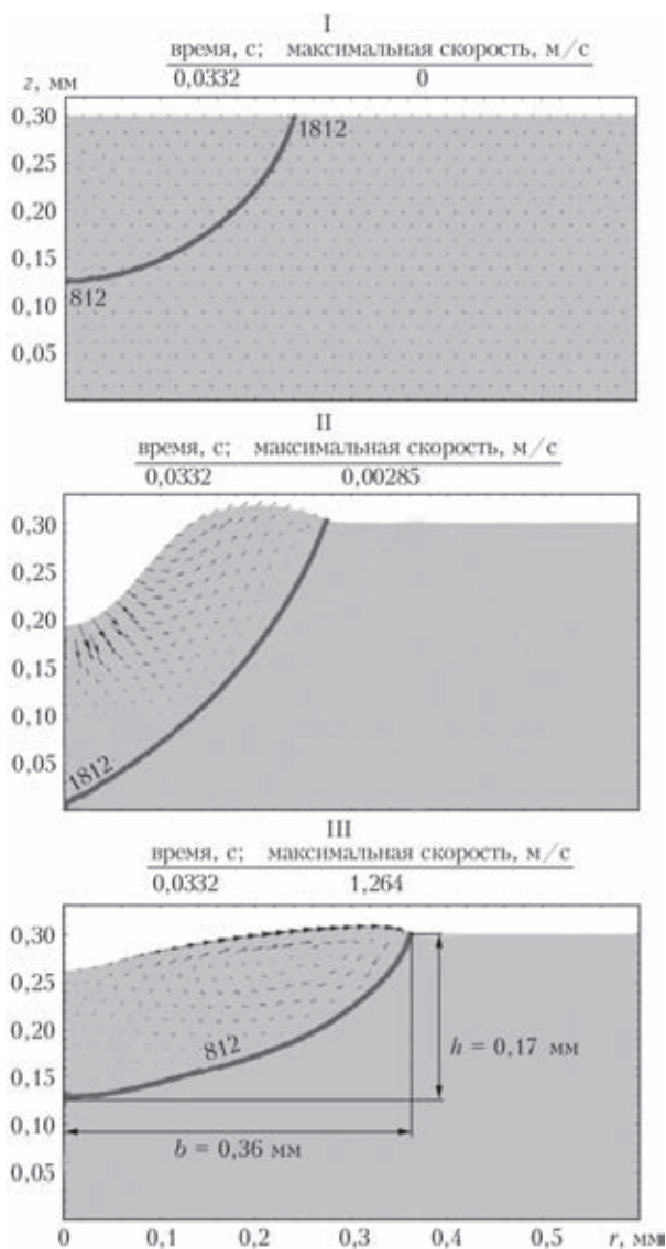
Рис. 7. Сравнительный анализ размеров и формы зоны проплавления, полученных с помощью различных моделей
