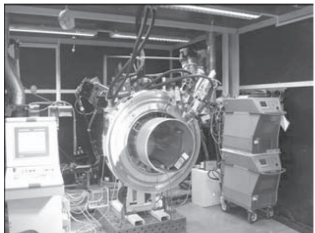
Рис. 5. Специализированная опытная установка для сварки трубопроводов
